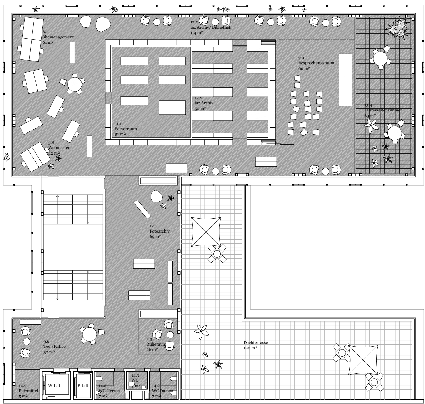
Grundriss 6. Obergeschoss 1:200
