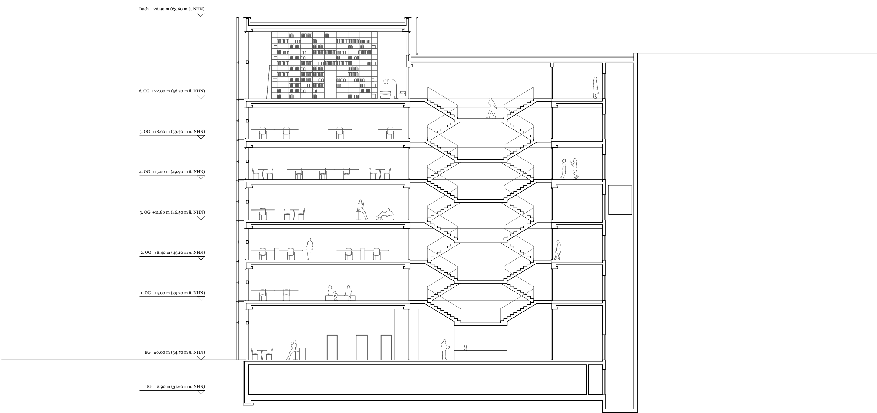
Schnitt A-A 1:200
