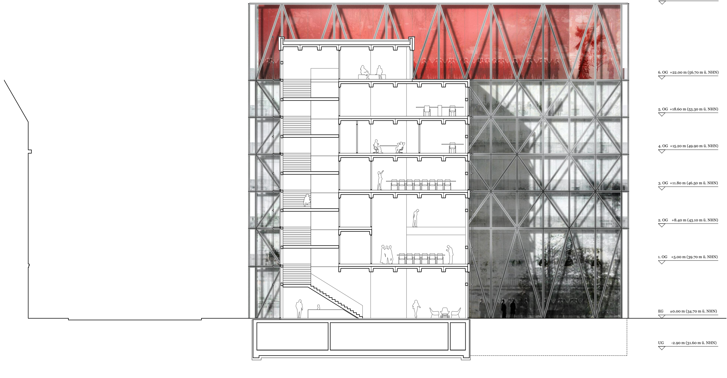
Schnitt B-B 1:200
