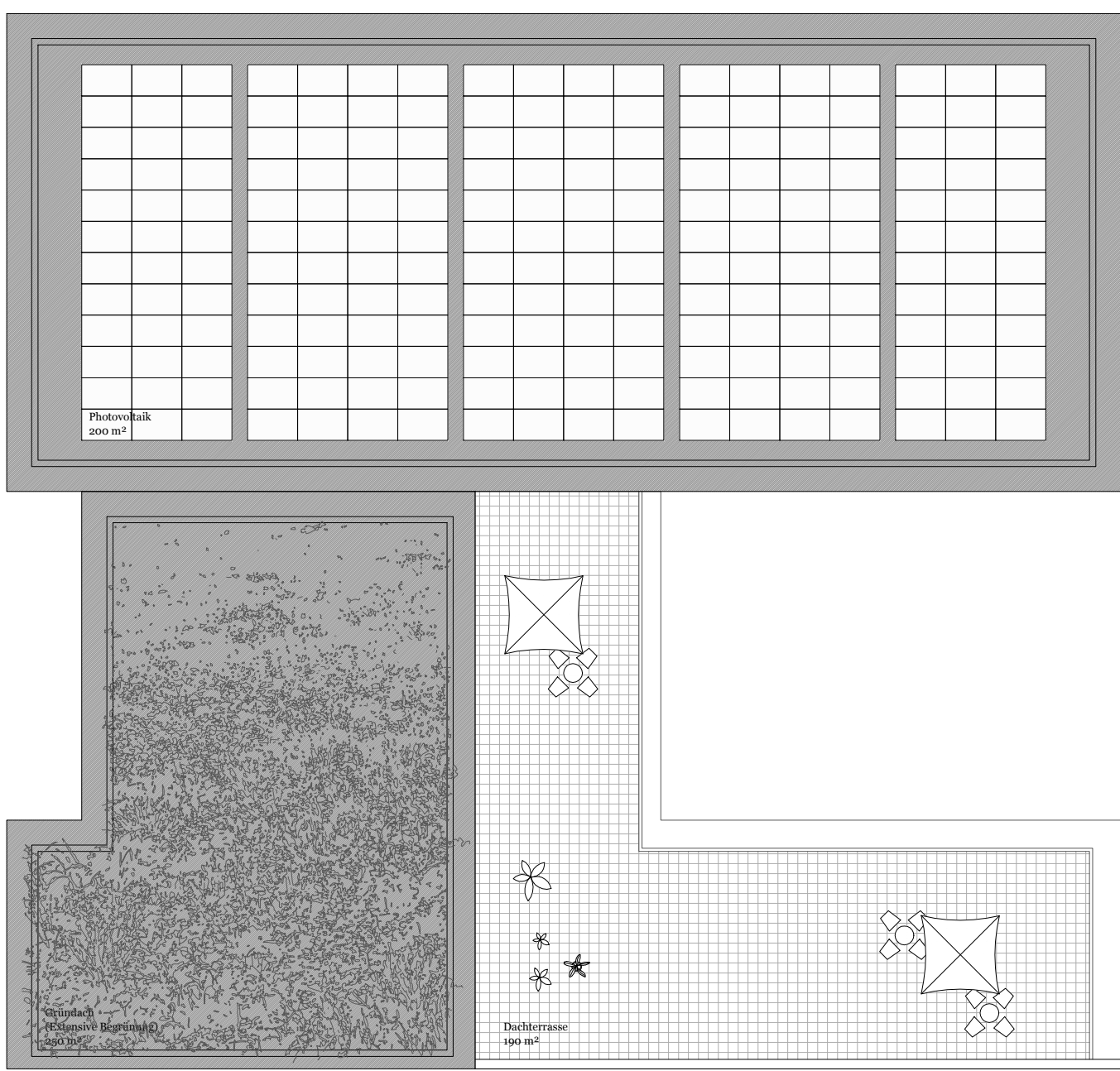
Dachaufsicht 1:200
