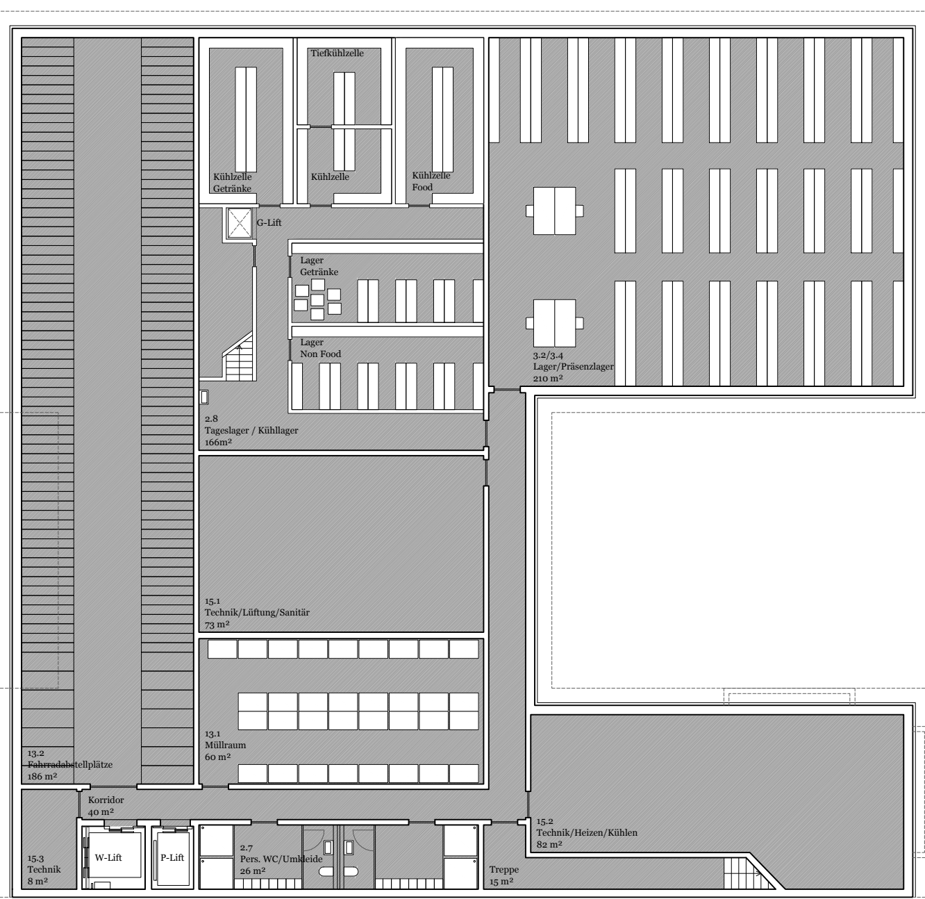
Grundriss Untergeschoss 1:200
